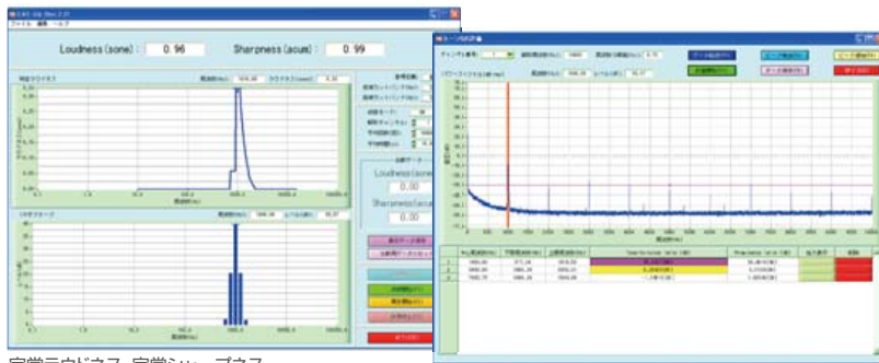
トーン性評価 (TNR, PR)
